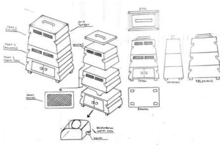
Gambar 3. Sketsa Pengembangan desain vermicomposting
